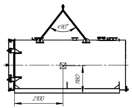
Схема строповки
